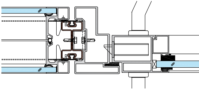
Horizontalschnitt Glastrennwand Lindner Life 125 mit Aluminiumzarge
